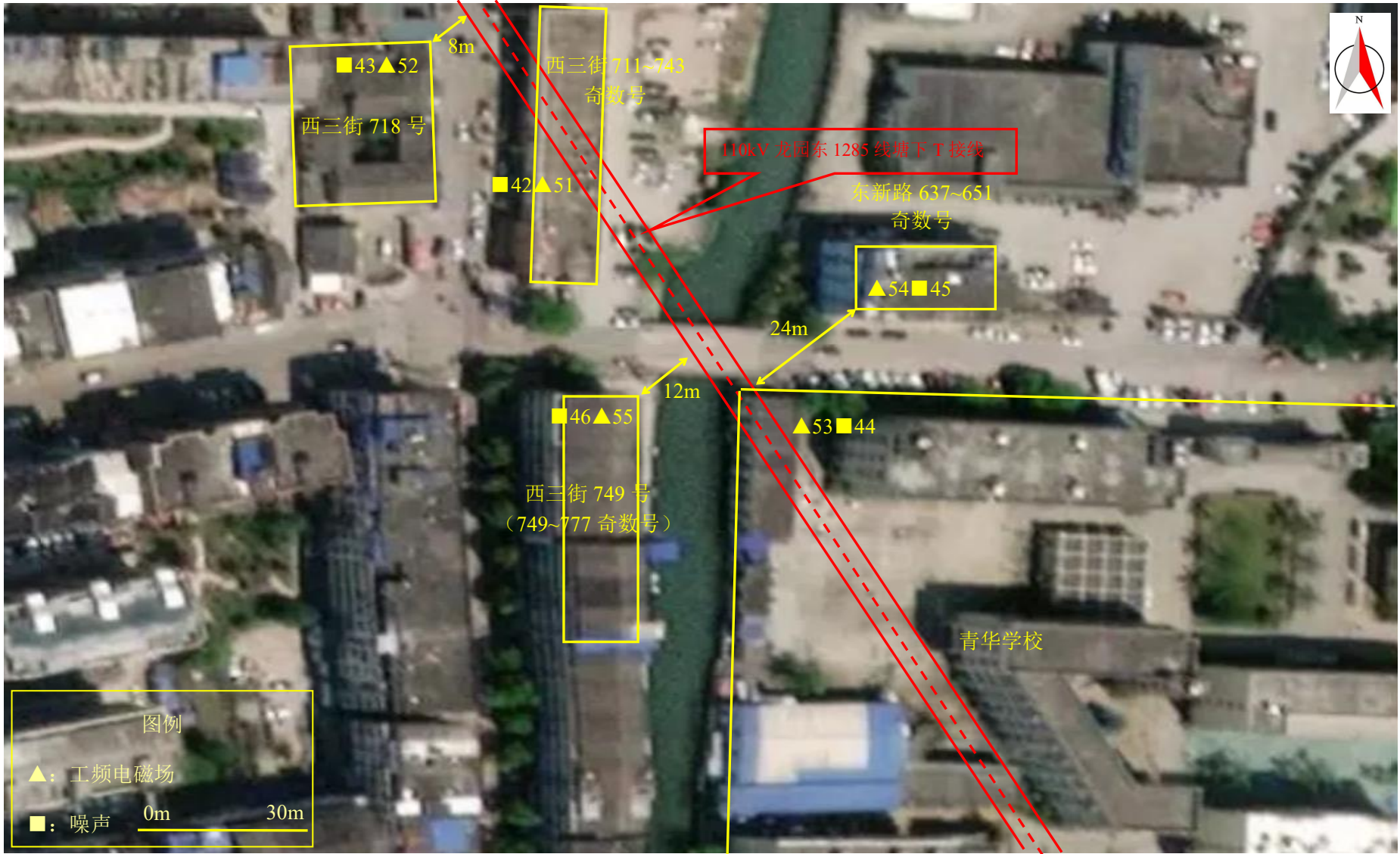
图 7-1 (9) 监测点位图
