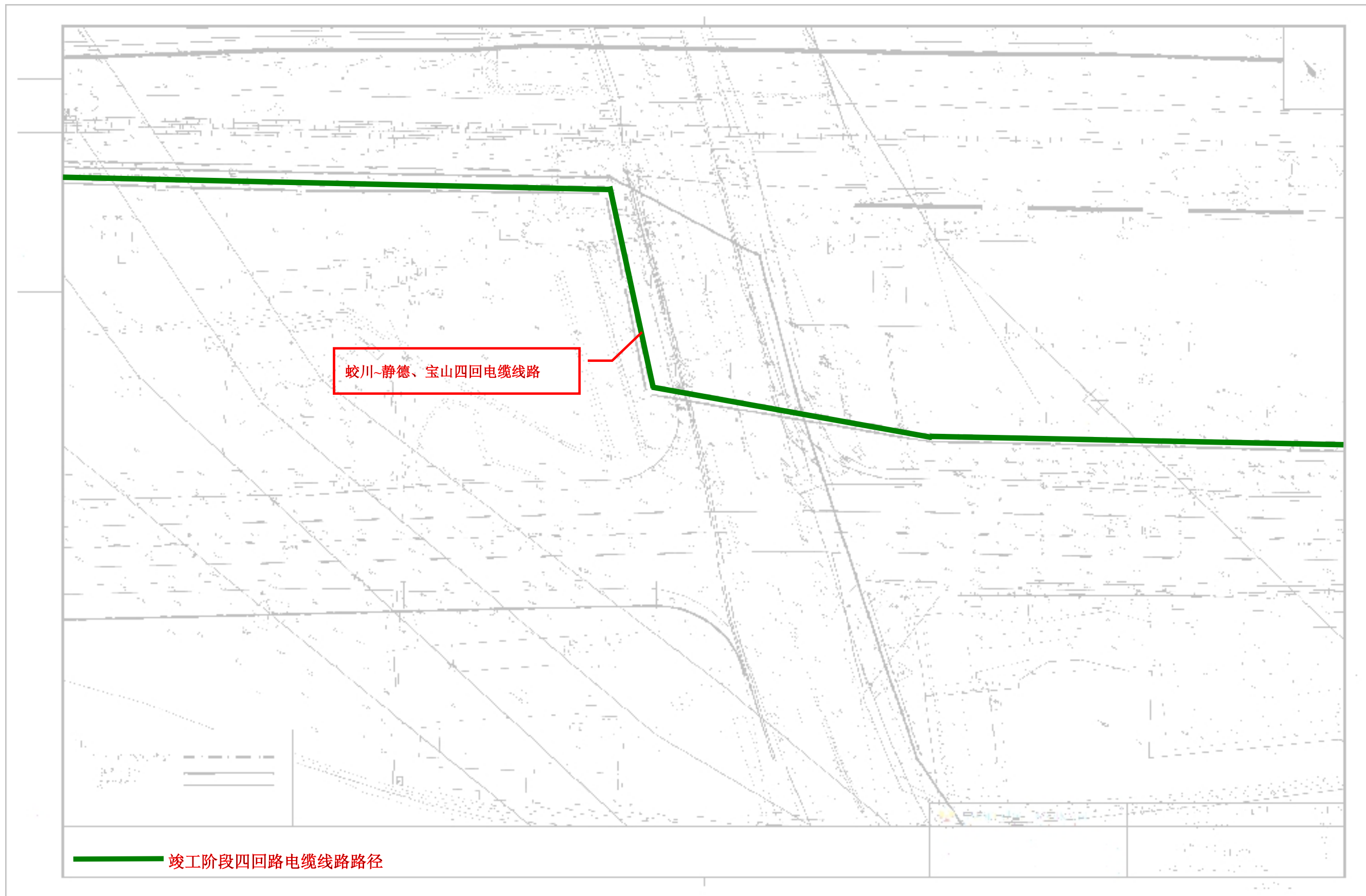
图 4-5 (2) 蛟川~宝山、静德改接新蛟川变 110kV 线路工程线路路径图
