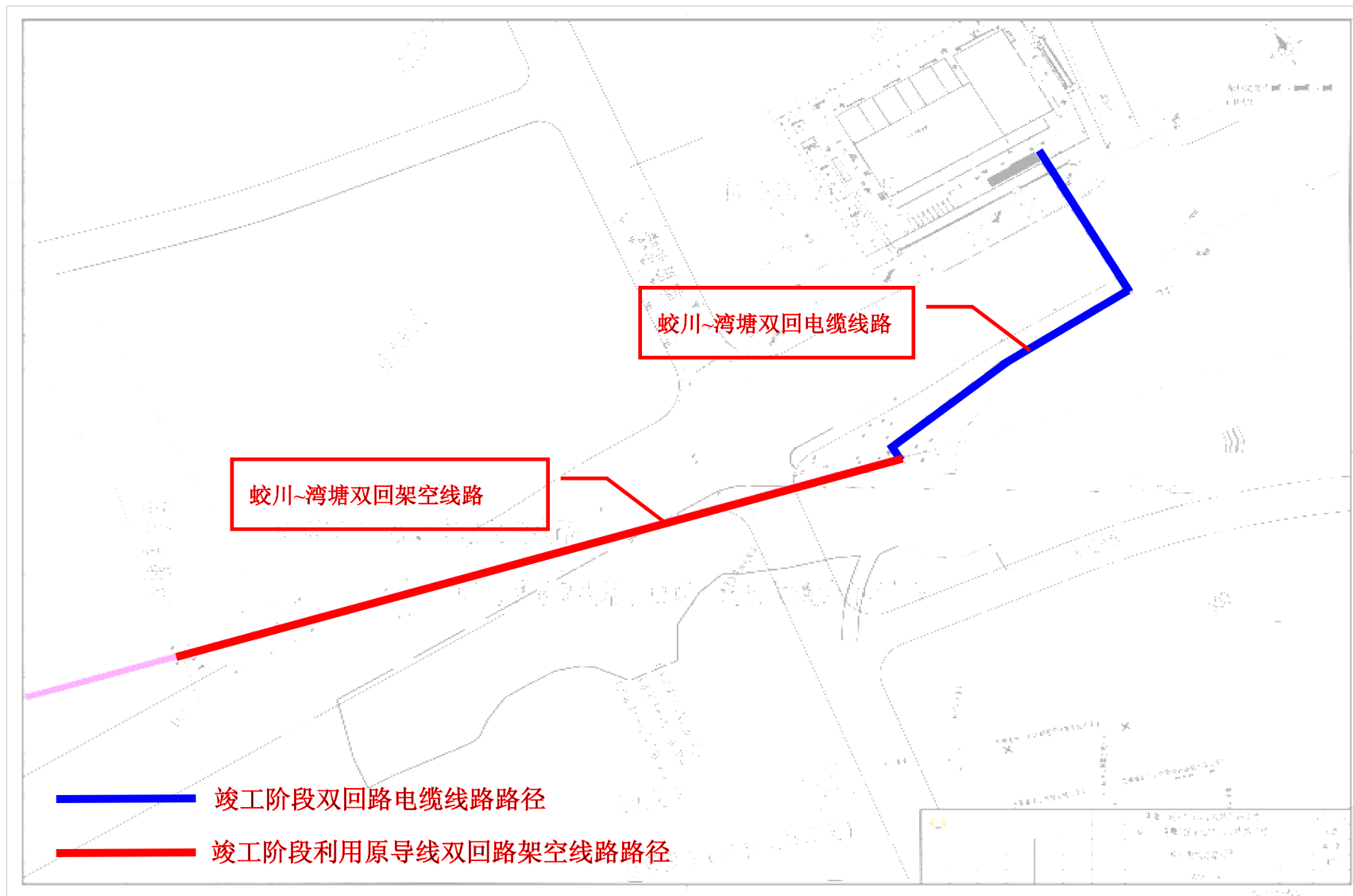
图 4-2 蛟川~湾塘改接新蛟川变 110kV 线路工程线路路径图
