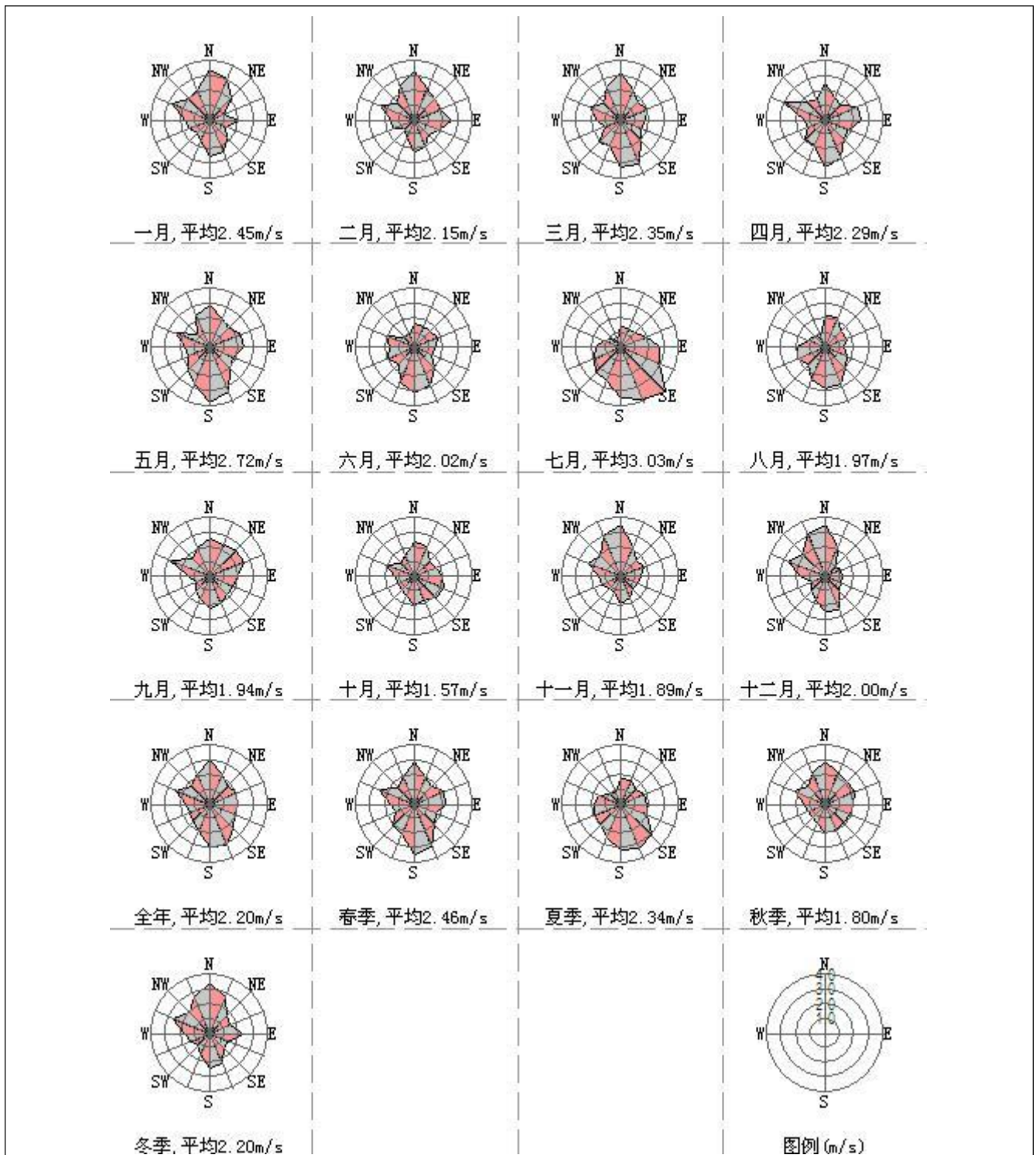
图 2-2 风速玫瑰图
