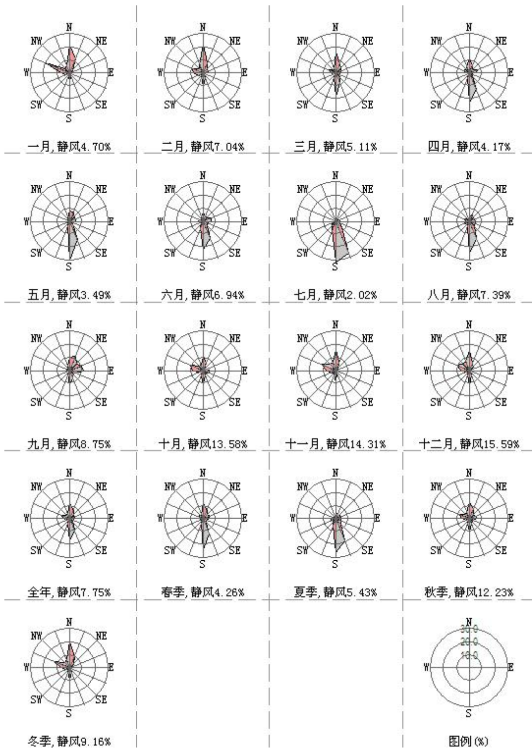
图 2-1 风向玫瑰图
