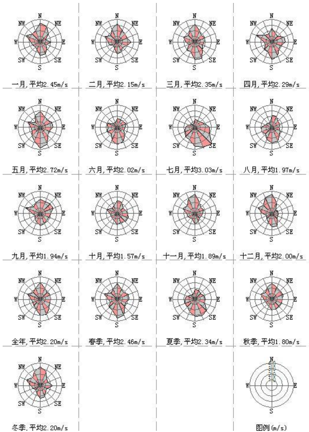
图 2-2 风速玫瑰图
