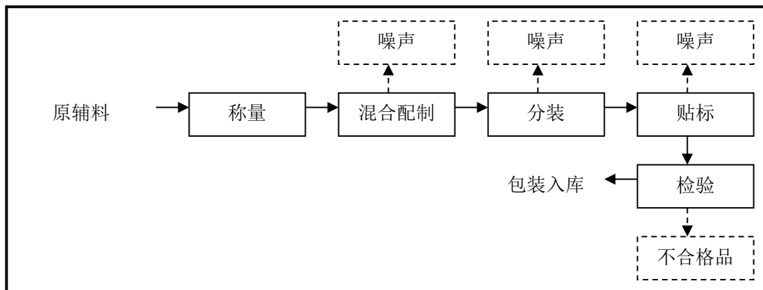
图 5-1 项目生产工艺及排污节点图
