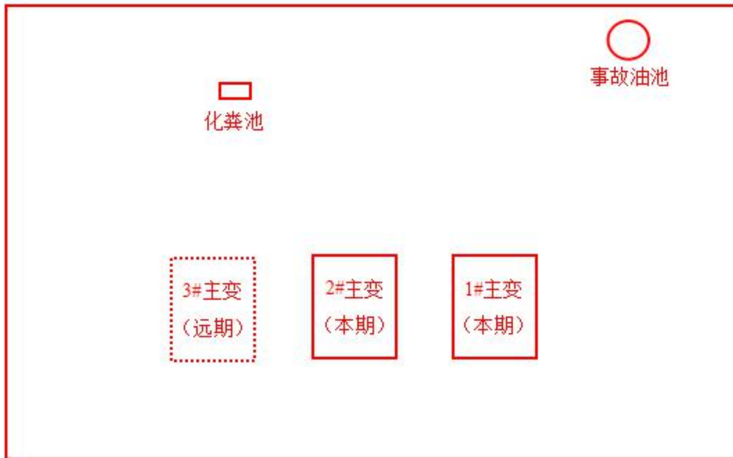
图 4-2 肯恩变平面布置示意图
