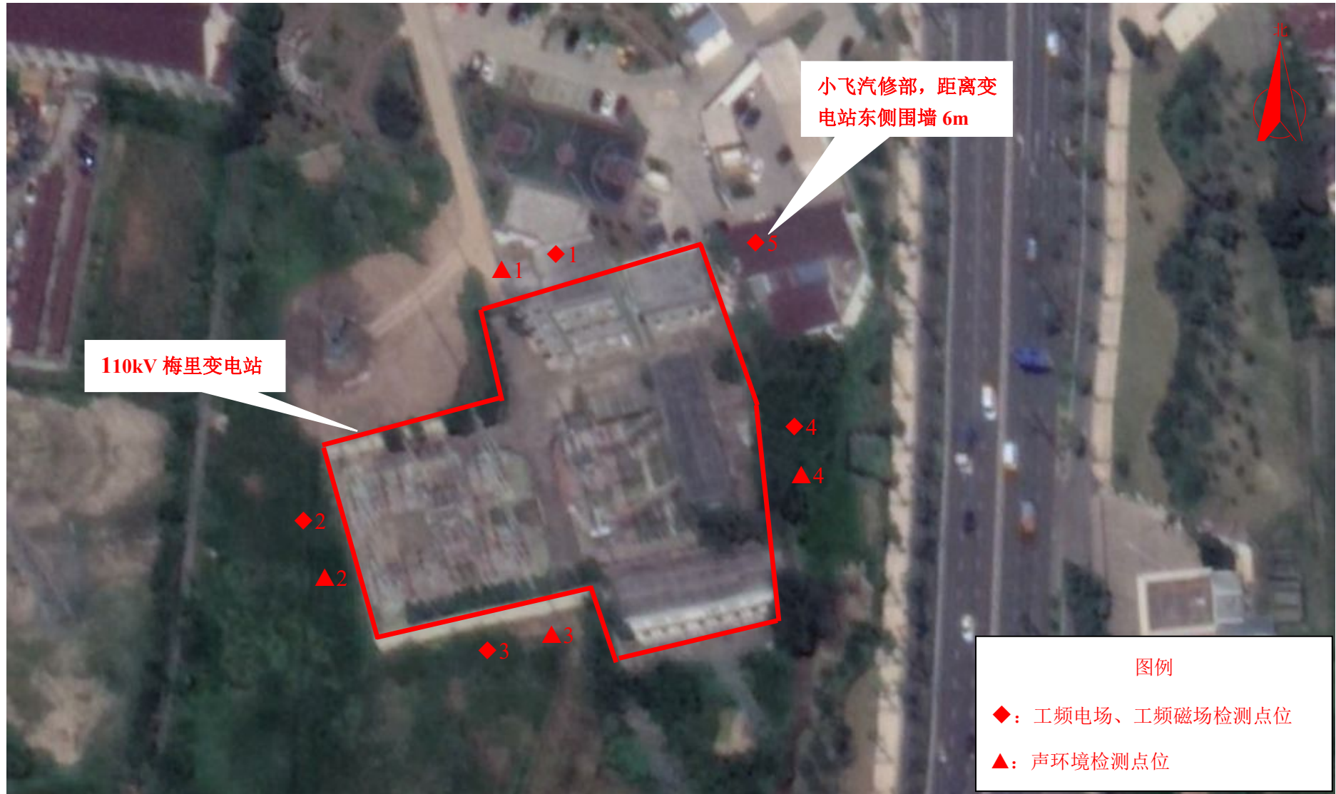
图 7-1 现场监测点位图 (110kV 梅里变电站工程)
