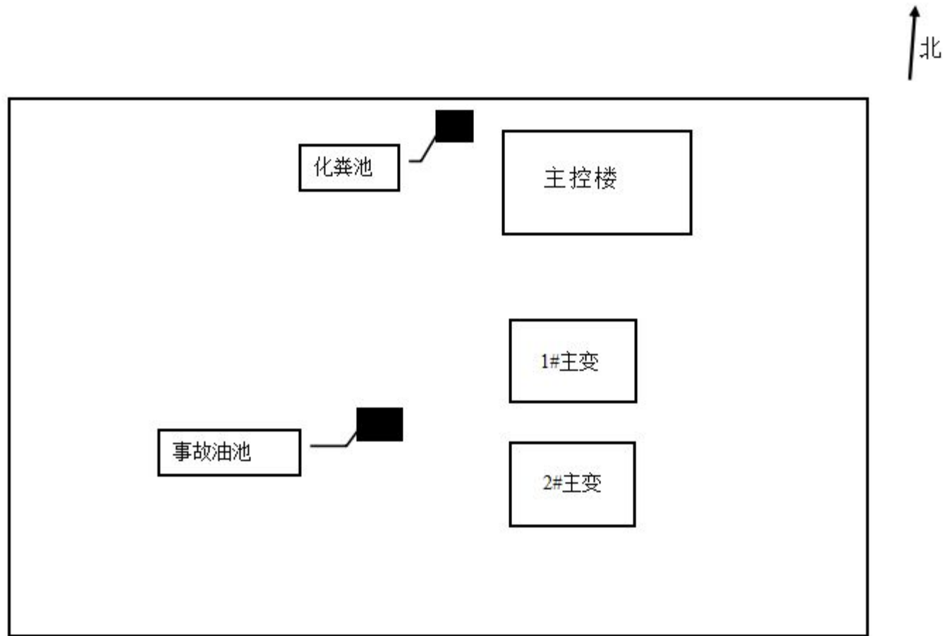
图 4-2 梅里变电站平面布置示意图
