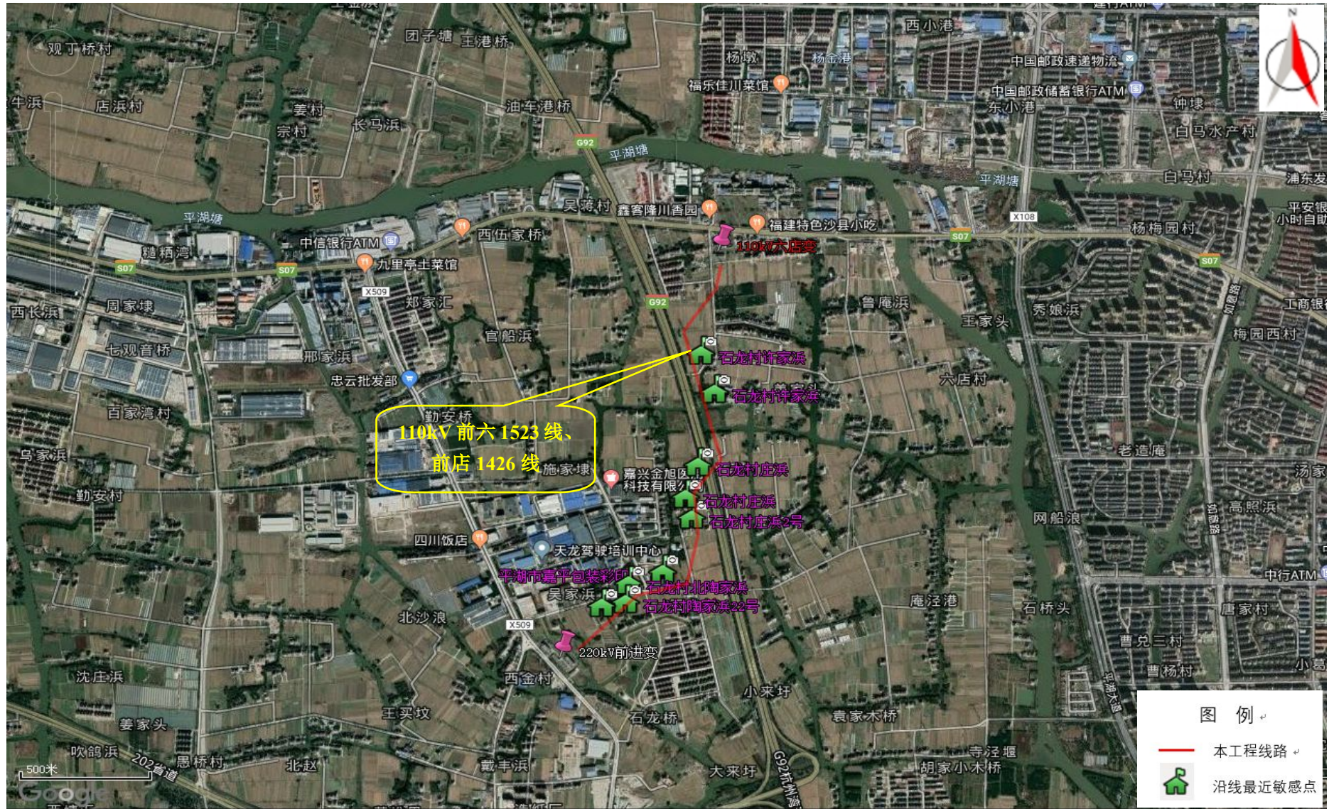
图 4-3 工程线路路径图（110kV 前六 1523 线、110kV 前店 1426 线）
