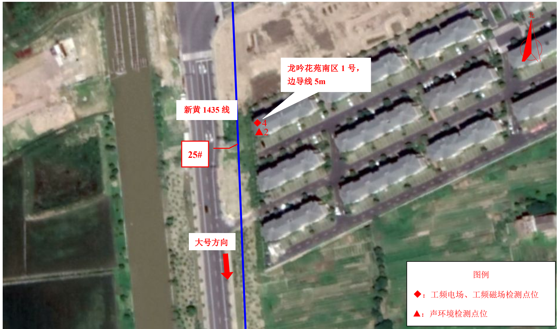
图 7-2 (3) 现场监测点位图 (110kV 黄姑输电线路工程)
