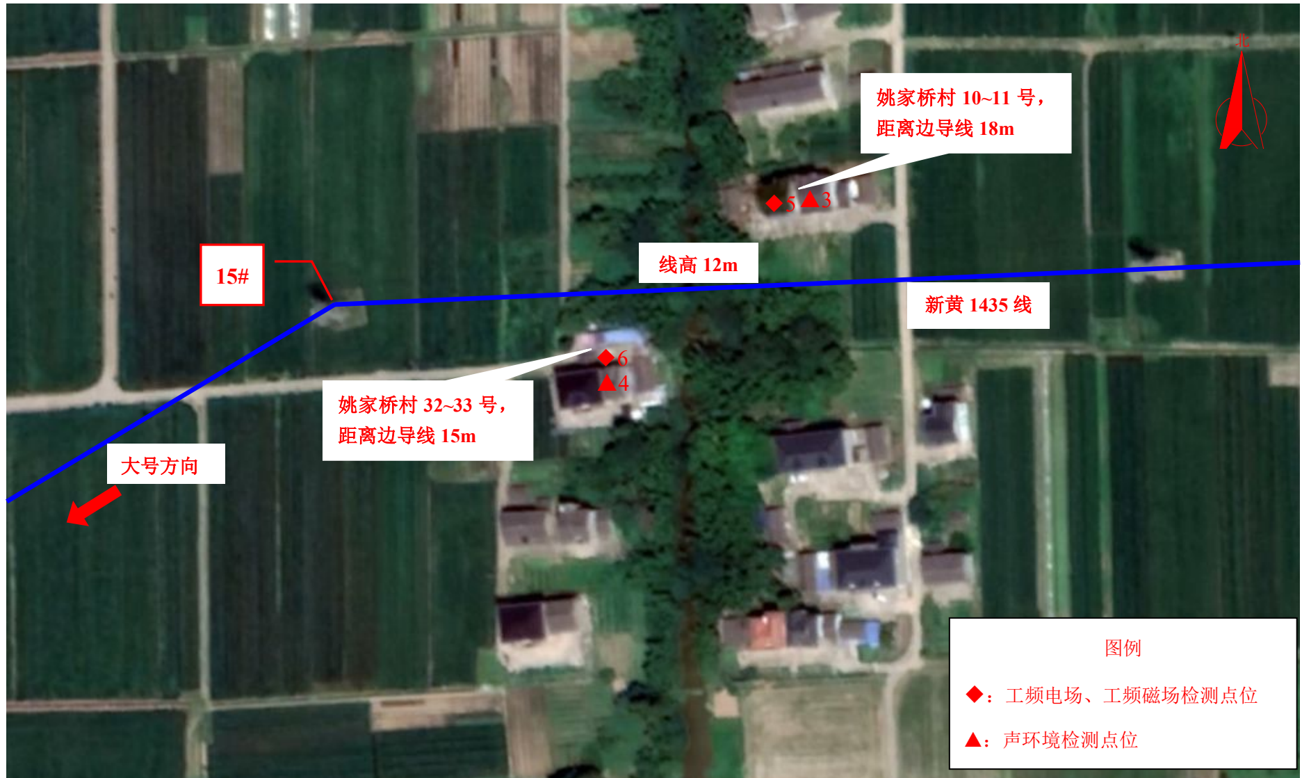
图 7-2 (4) 现场监测点位图 (110kV 黄姑输电线路工程)
