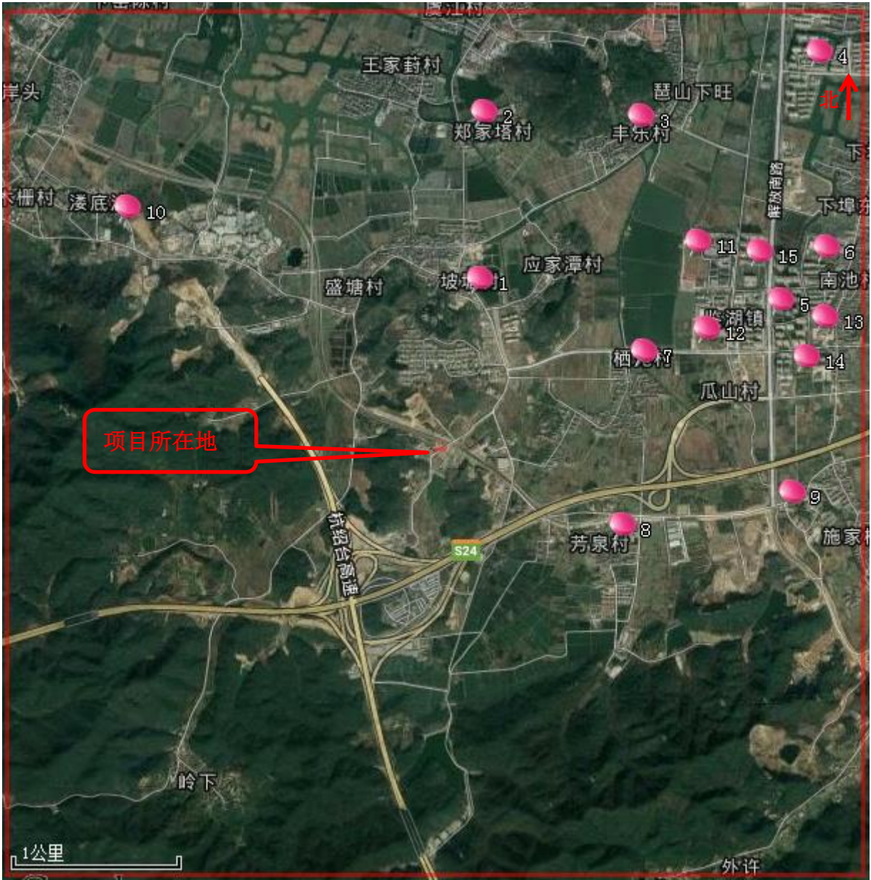
图 3.2 大气评价范围及评价范围内主要敏感点示意图（边长 5 km）
