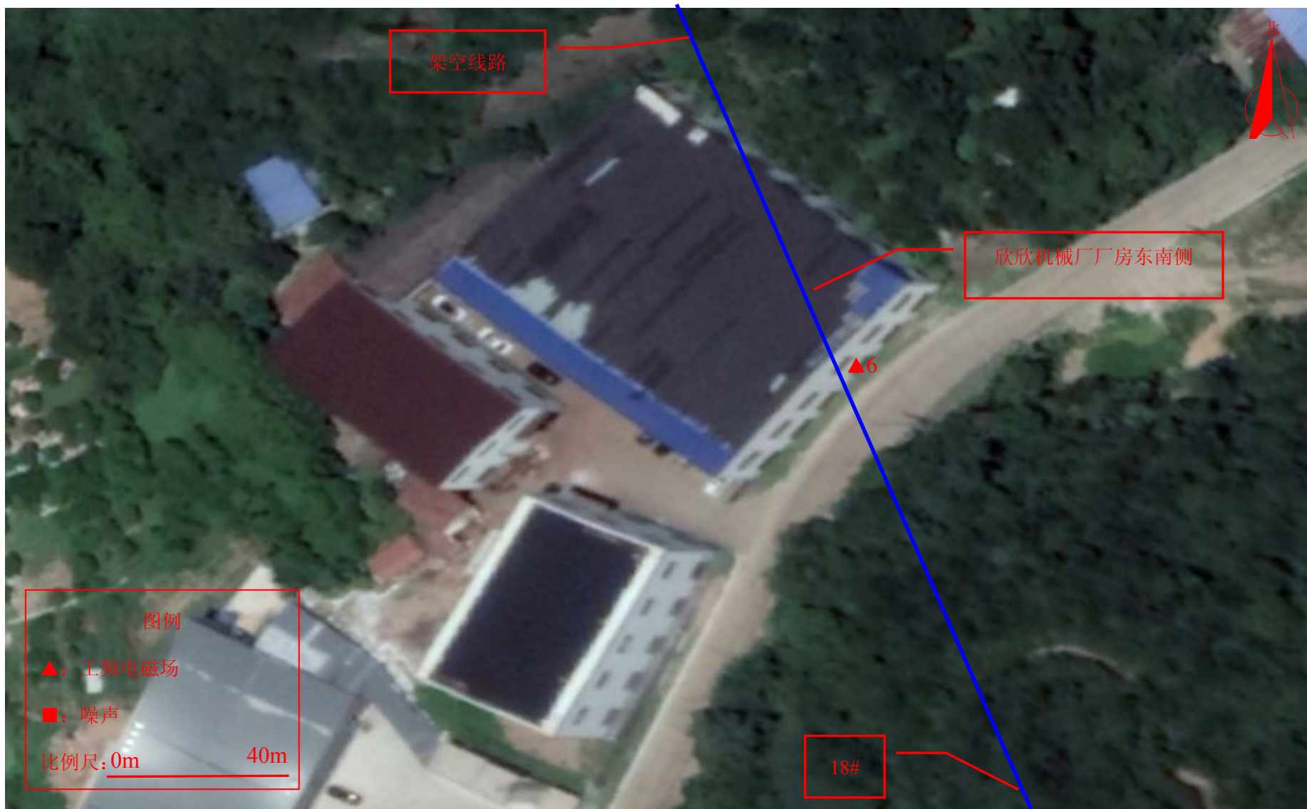
图 7-1 (3) 现场监测点位图
