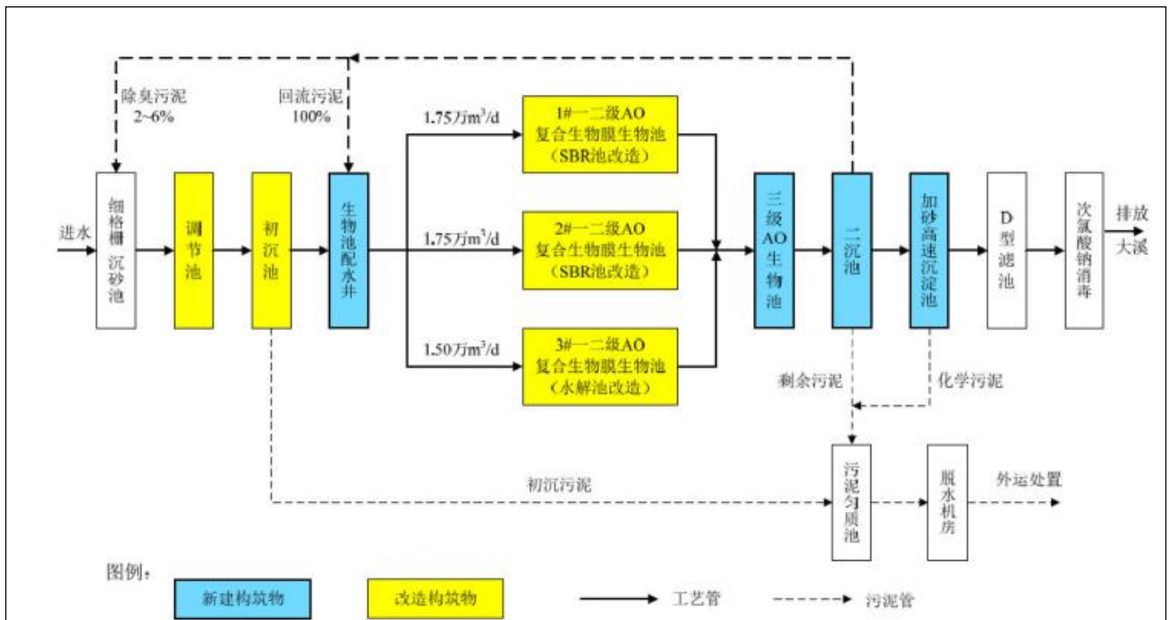
图 2-1 水阁污水处理厂污水处理工艺流程图
